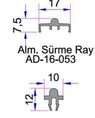
Alm. Sürme Ray AD16-053
