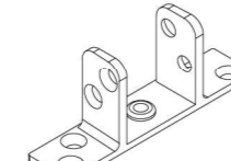
Kanat İçi Orta Kayıt Bağlantı Takozu 21283.0000.0.2
