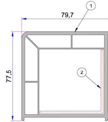
Kısa Bağ Profili P.A.099.5003.600
