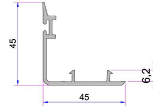
Süper Kanat Arka Kapama Profili P.A.222.5700.600
