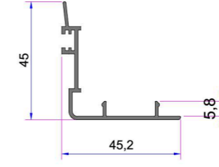
Alm. Süper Kanat Arka Kapama Profili AD16-032
