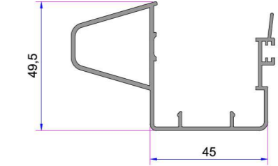
Alm. Kanat Arka Kapama Griyaj Profili Kalıp Yeni Yapılacak
