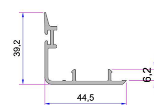
Kanat Arka Kapama Profili P.A.222.5708.600
