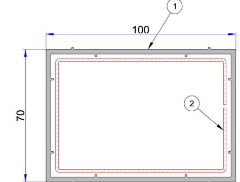
Alm. Çift Ray Adaptörü AD16-011
