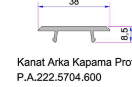
Alm. Kanat Arka Kapama Griyaj Profili Kalıp Yeni Yapılacak
