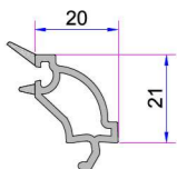
4mm Tek Cam Çıtası P.A.101.4102.600.0.HC
