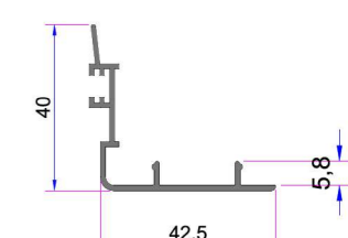
Alm. Kanat Arka Kapama Profili AD16-031
