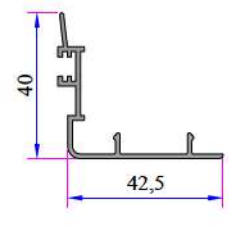
Alm. Kanat Arka Kapama 16031.601.5.11.9016
