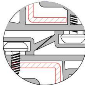
Sürme Kanat Arka Kapama Montajı
