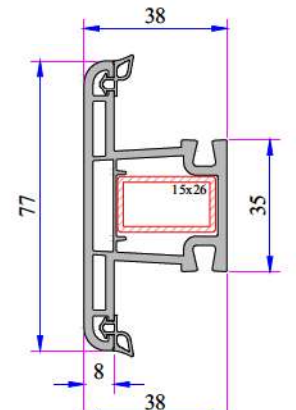
Kanat İçi Orta Kayıt Profili P.A.222.3201.600.0.BC.01
