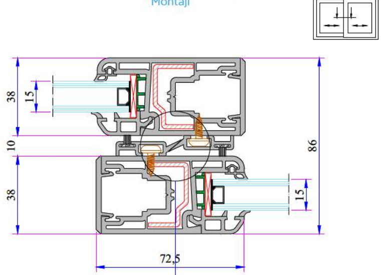
Sürme Kanat Alm. Arka Kapama Montajı
