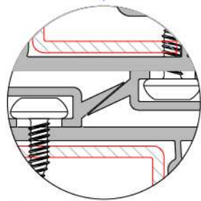
Süper Sürme Kanat Arka Kapama Montajı
