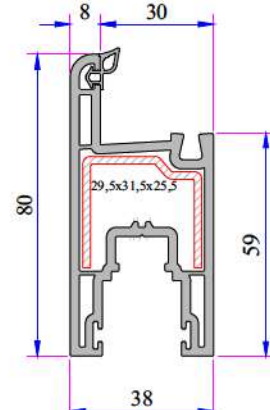
Süper Sürme Kanat Profili P.A.222.2304.600.0.BC.01
