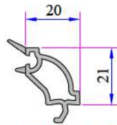
Tek Cam Çıtası 4-6mm P.A.101.4002.600.0.HC
