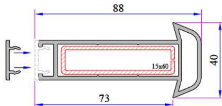
Üniversal Kalın Bağ Profili P.A.058.5000.600.0.19
