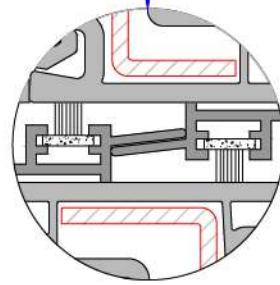
Sürme Kanat Alm. Arka Kapama Montajı
