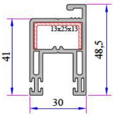
Sürme Sineklik Kanat Profili P.A.242.2305.600.0.00.03
