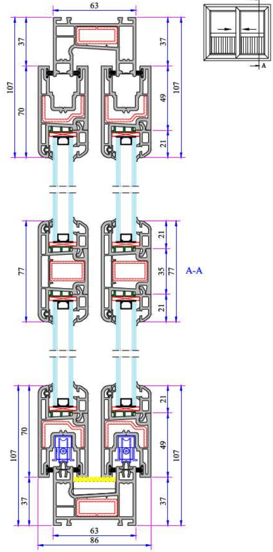
Kanat İçi Orta Kayıt Montaj Detayı
