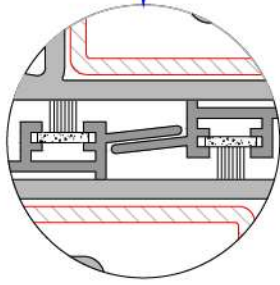
Süper Sürme Kanat Alm. Arka Kapama Montajı
