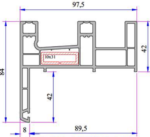
Sürme Pervazlı Sineklik Kasa Profili P.A.222.1109.600.0.00.01
