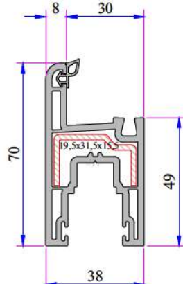
Sürme Kanat Profili P.A.222.2300.600.0.BC.01
