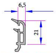
Çift Cam Çıtası 17mm P.A.532.4500.600.0.HC
