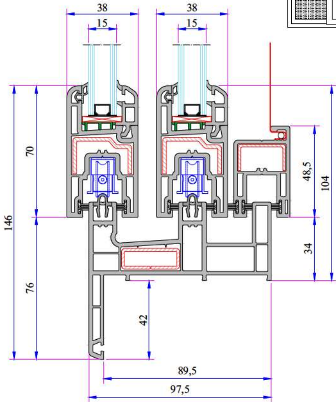
Sürme Pervazlı Sineklik Kasa - Sürme Kanat Montaj Detayı
