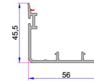
PVC Kanat Ara Bindirme Contası P.A.232.5700.600
