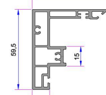
Üç Bölmeli Sürme Alm. Orta Kayıt Profili Profil YENİ Yapılacak
