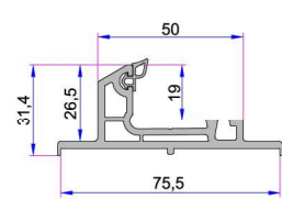
Çift Ray Adaptör Profili P.A.232.5800.600
