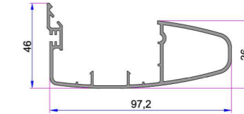
Alm. Kanat Arka Kapama Griyaj Profili 16028.601.5.2.0.9016
