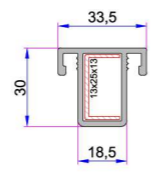
Sürme Sineklik Orta Kayıt Profili P.A.242.3200.600.0.00.19
