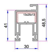
Sürme Sineklik Kanat Profili P.A.242.2305.600.0.00.19
