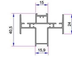
Alm. Kulaklı Çift Kanat Adaptörü Profil YENİ Yapılacak
