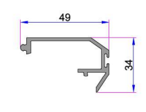
Alm. Kasa Kanal Kapama Profili AD 16 - 013
